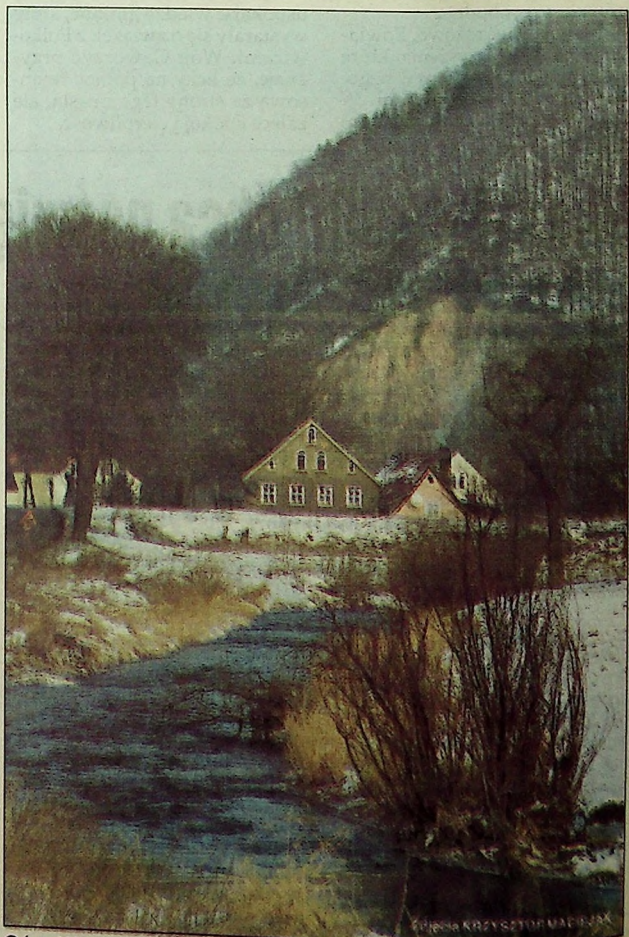
Góra Wielistawska nad Kaczawą, przykład dawnego wulkanizmu.
