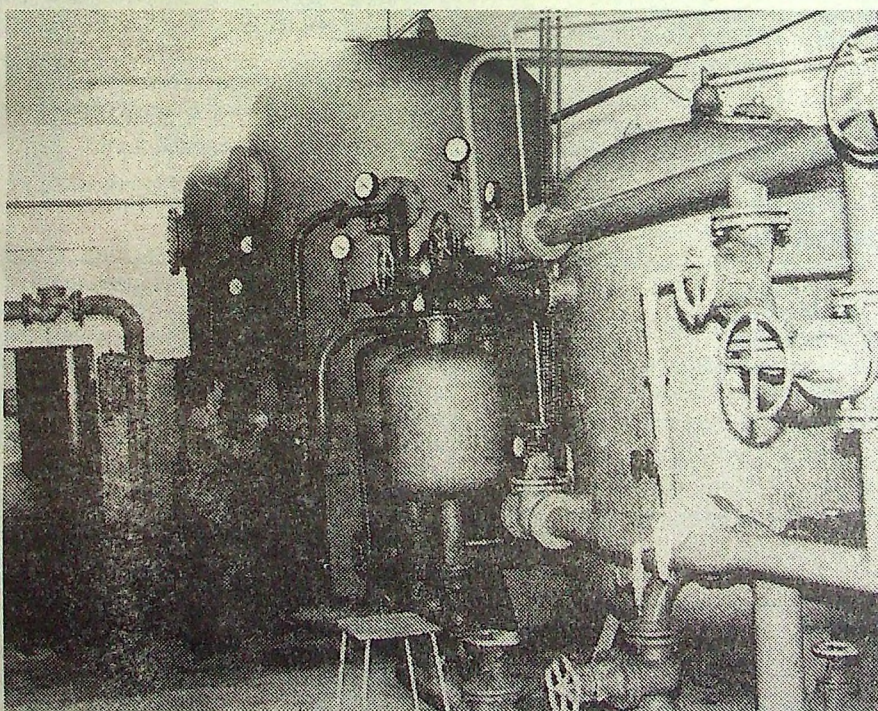
Budowę stacji uzdatniania wody w Przemkowie zakończono w 1995 roku, ale pełną moc produkcyjną osiągnięto w 1996 roku.
