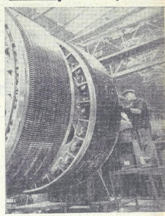
ЛЕНИНГРАД. Коллектив производственного объединения «Электросила» изготавливает три уникальных гребных двигателя для атомного ледокола «Сибирь», который сооружается на главном стапеле Балтийского судостроительного завода имени С. Орджоникидзе. Электромашиностроители, поддерживая инициативу балтийцев, делают все возможное, чтобы обеспечить спуск на воду нового ледокола-исполнителя к открытию XXV съезда КПСС.
