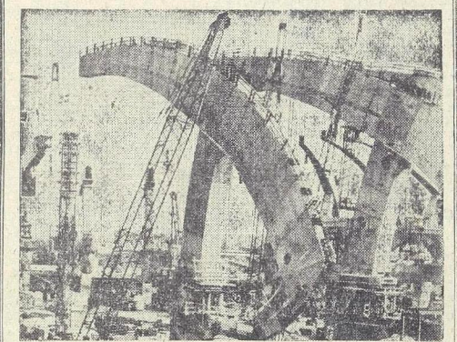
КАНАДА. Монреаль готовится к приему участников и гостей Олимпиады-76. Строится Олимпийская деревня. Растут спортивные сооружения. На снимке: на строительстве олимпийского стадиона. Фото АПА—ТАСС.
