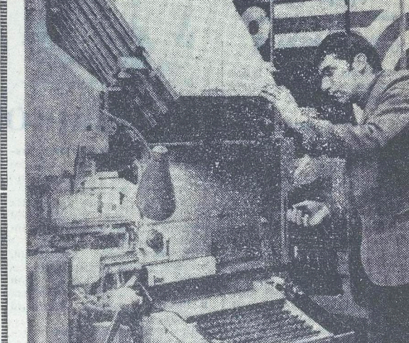
На снимке: машина Н-140 из унифицированного ряда наборных строкотайных машин «Россия». Фото О. Лазаренко.
