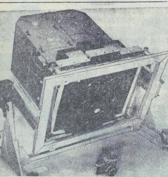
ГДР. Экипаж космического корабля «Союз-22» провел съемки земной поверхности с помощью многозональной фотоаппаратуры.
