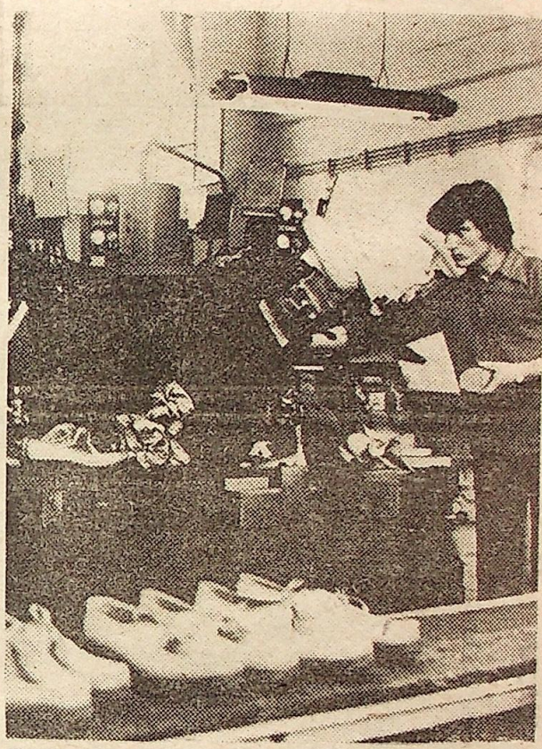
Zakład Obuwia „Odra” w Złotoryi wyprodukował w tym roku już 1 mln 54 tys. par poszukiwanego na rynku obuwia tekstylnego. Na zdjęciu: Stanisław Haponik przy wtryskiwaniu podeszew.
