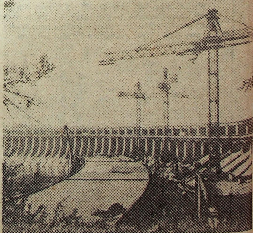
To już historia. Budowa „Dnieprogesu-2”. Dziś elektrownia jest włączona do systemu energetycznego.
