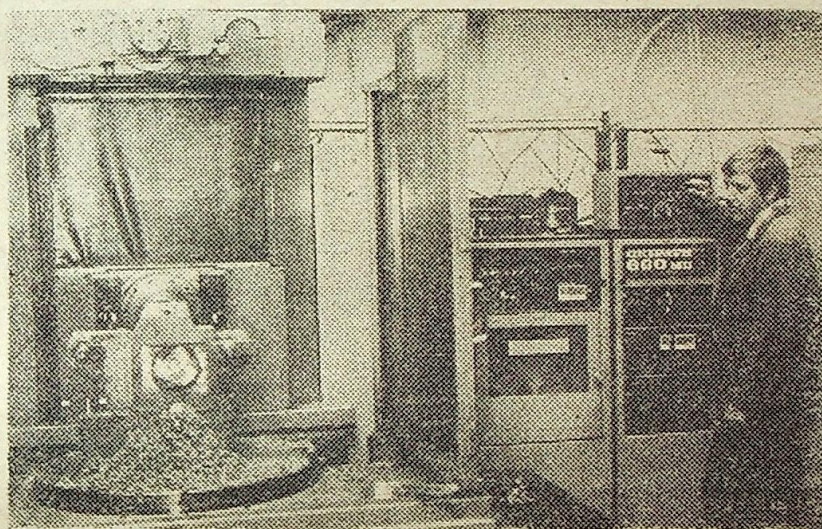
Chocianowska Fabryka Automatów dysponuje nowoczesnymi urządzeniami technicznymi. I tak np. w centrum obróbczym zainstalowana została aparatura produkcji japońskiej OKIPATH 660 M II firmy Mitsui Seiki. Bronisław Byra przy tej właśnie aparaturze w czasie obróbki tylnego mostu wiertarki hydraulicznej.
