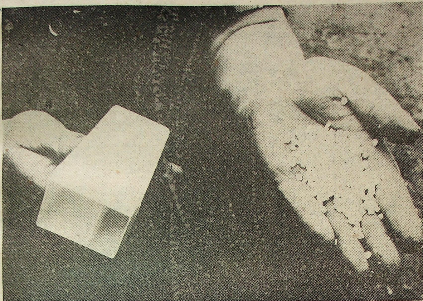
Wtryskarka zamienia granulat w etui na szczotkę i pastę do zębów.
