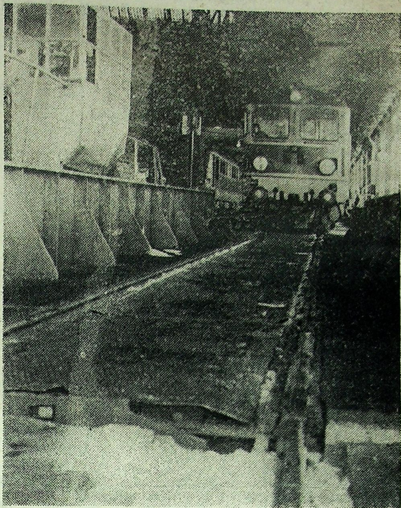
Biała plama na pierwszym planie to beton porwany kołami wykolejonych lokomotyw, które zjeżdżają z przesuwni. Powód? Różne szerokości torów...
