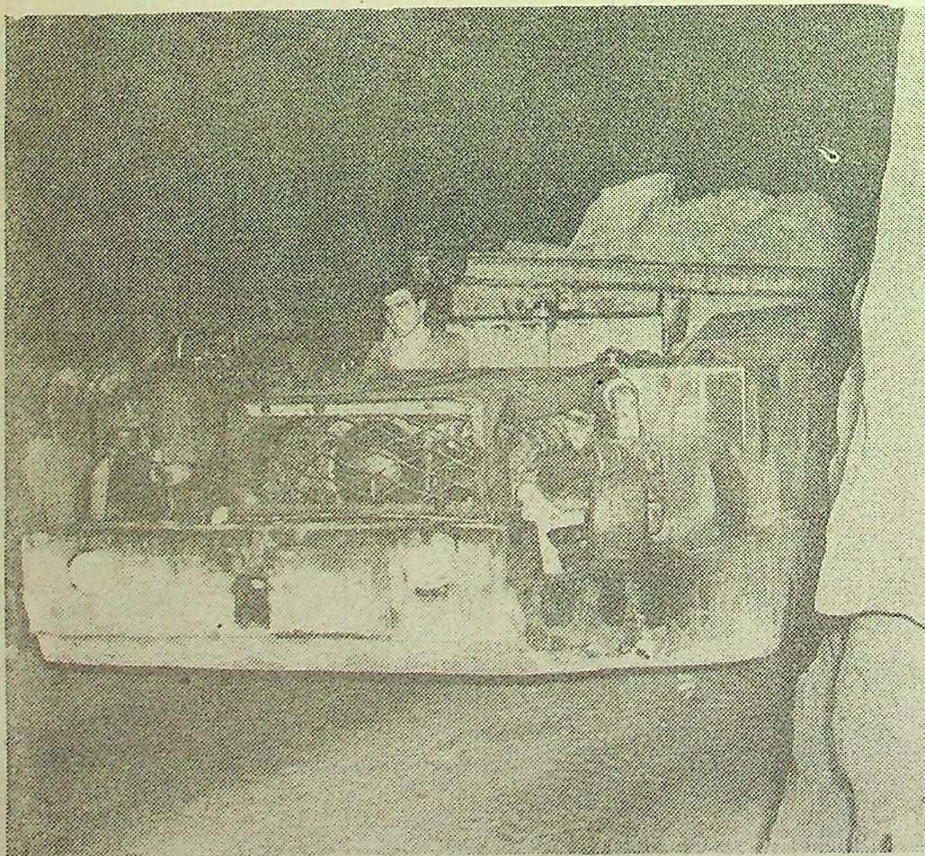
Produkowane dziś wozы odstawcze zabierają jednorazowo 15 ton urubku. Już wkrótce zakład przystąpi do montażu maszyn 35-tonowych.
