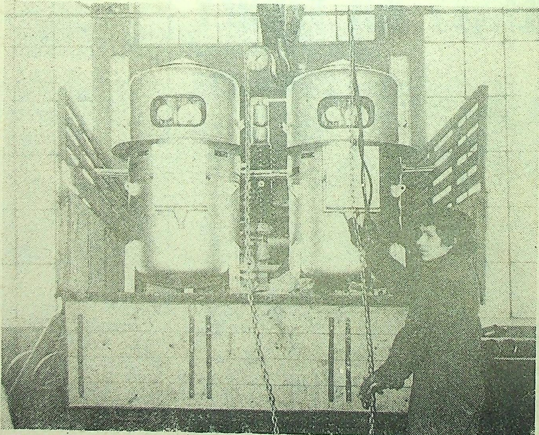
W warsztacie mechanicznym wykonuje się wiele urządzeń dla potrzeb zakładu. Ukończono właśnie montaż dwóch kompresorów.
