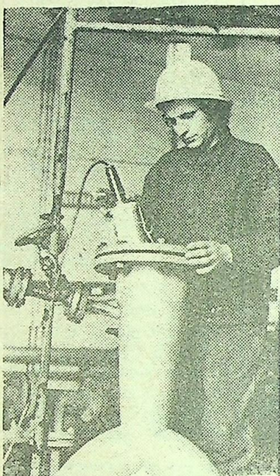
Stanisław Borsuk kontroluje układ krystalizacji soli fosforowych.
