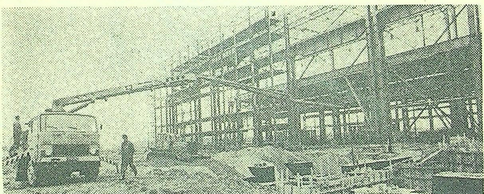
Roboty betoniarskie w hali pieców wykonuje Poznańskie Przedsiębiorstwo Budownictwa Przemysłowego nr 1.
