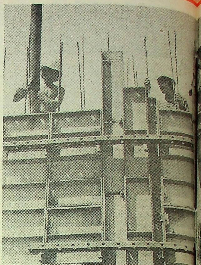
Eksploatowane od lipca 1975 roku szalunki „Neo” znacząco przyspieszają stawianie ścian. Henryk Gryglel, Henryk Kulski i szard Cegielnik podczas wlewania betonu.
