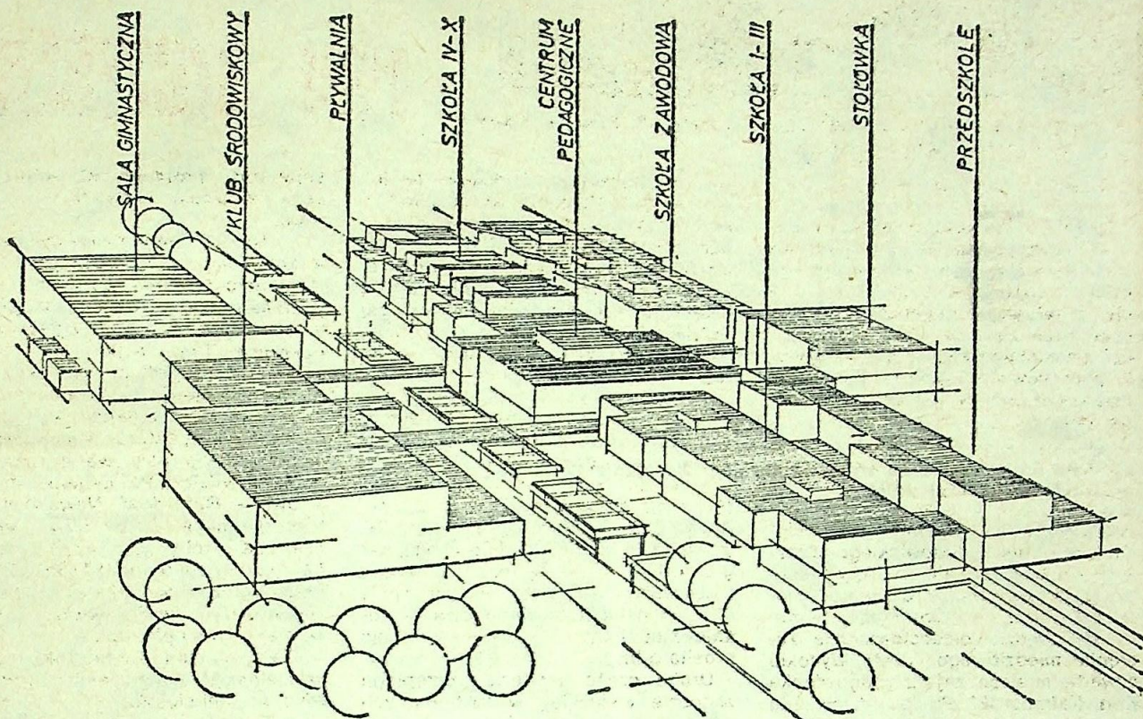
Szkic rozwiązania funkcjonalnego „szkoły przyszłości” zaprojektowanej przez zespół architektów ze Szczecina, kierowany przez Jana Czuchnickiego. Projekt uzyskał jedną z głównych nagród w konkursie ogłoszonym przez SARP i nagrodę ministra oświaty i wychowania za koncepcję pedagogiczną.
