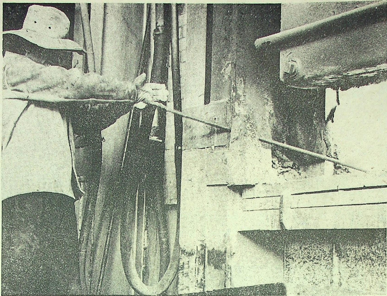
Ten piec anodowy ruszył 31 sierpnia. Andrzej Łukasiewicz pobiera próbkę miedzi.
