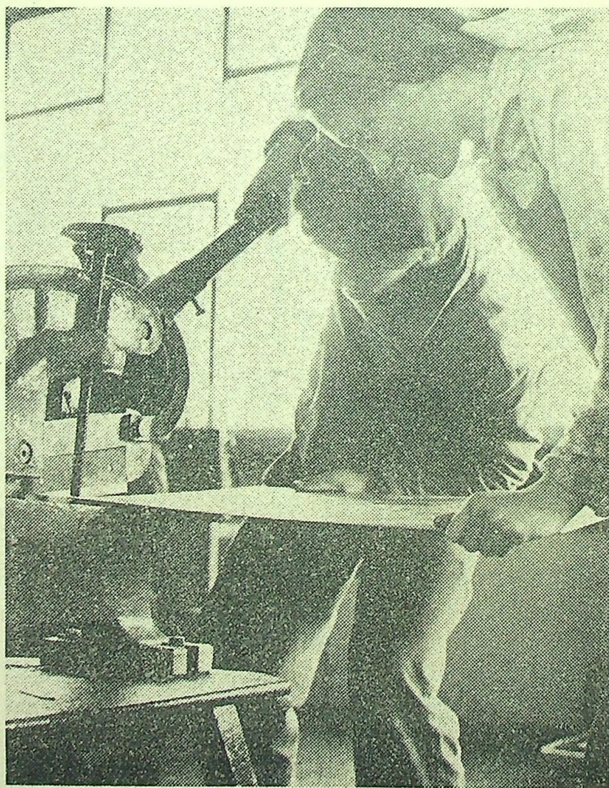
Powstaje kolejna elektryczna szafka rozdzielcza.
