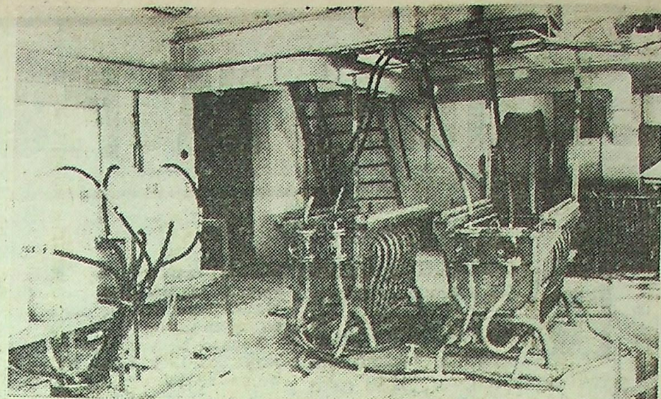
Aparatura pilotująca do elektrolitycznego wydzielania miedzi i regeneracji czynnika ługującego, zainstalowana w Zakładach Doświadczalnych HYDROMECH w Kowarach.
