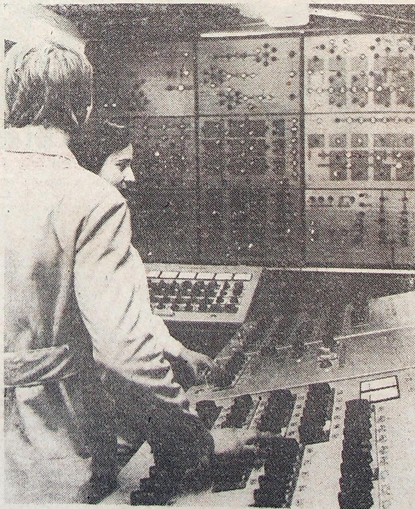
Wytwórnia pasz w Ujeździe Górnym — jedna z czternastu tego ty- pu w kraju — zatrudnia 110 ludzi. Ale samą produkcję mogłoby te- oretycznie robić dwoje ludzi sterując całym procesem technologicz- nym przy pomocy tych pulpów. Na zdjęciu operatorzy: Helena Ży- lińska i Jerzy Golec.
