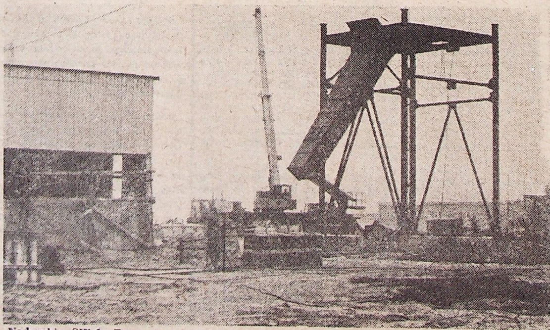
Nadszybie SW-3. Trwa w przyspieszonym tempie budowa konstrukcji tymczasowej wieży wyciągowej. Operacja jest bardzo pracochłonna i wymaga zachowania szczególnej ostrożności.
