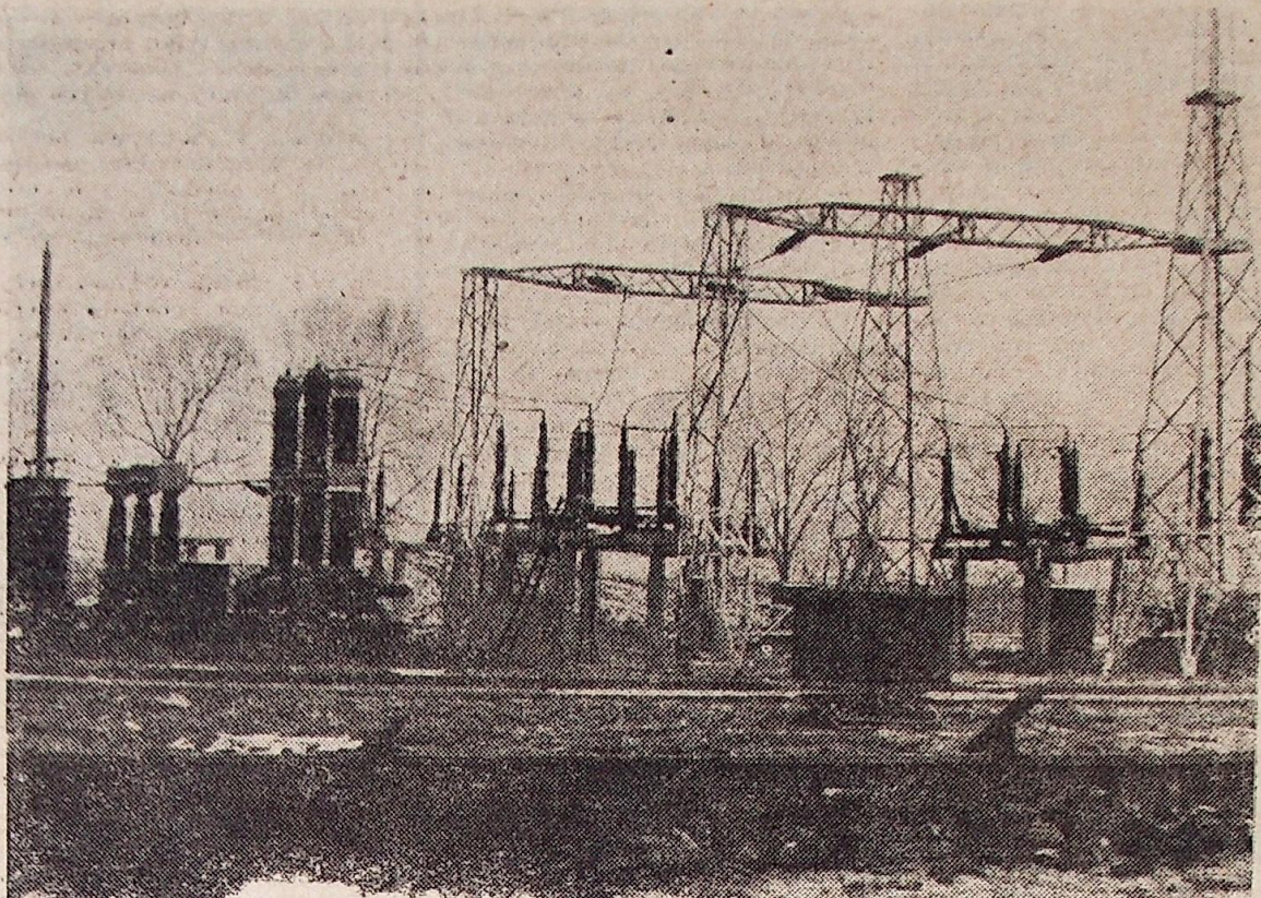
Główna stacja transformatorowa o mocy 110 KW rozpoczyna pracę na terenie szybu SW-3 o blisko 4 miesiące wcześniej niż pierwotnie zakładano. Dzięki zobowiązaniu załogi wrocławskiego „Elektromontażu” można będzie szybciej rozpocząć mrożenie i głębenie szybów.
