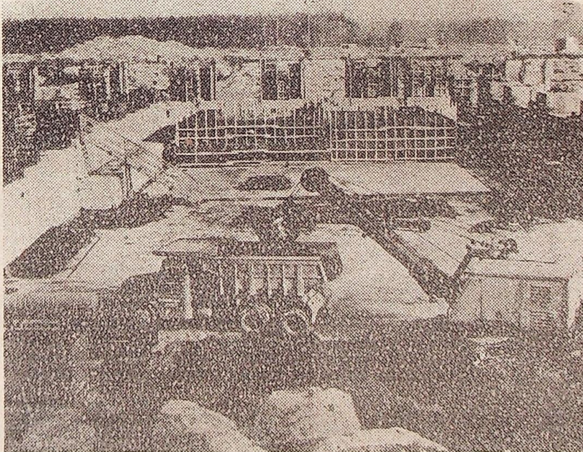
Od kilku lat przeżywamy prawdziwie zmasowany atak budowniczych na obiekty energetyczne. Elektrownia „Opole” jest jedną z kilku wznoszonych obecnie w naszym kraju. Na zdjęciu: betonowanie i zbrojenie fundamentów. Fot. CAF — Okeński
