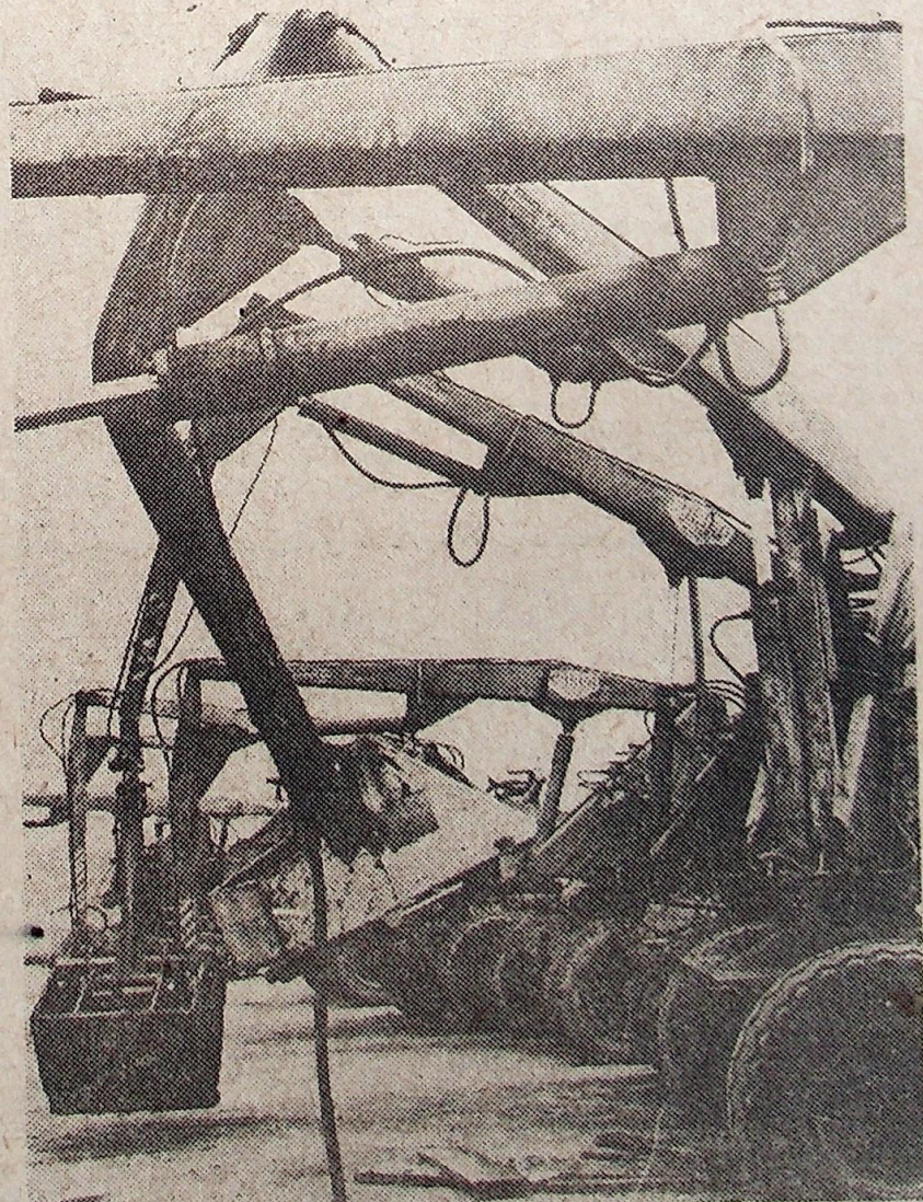
Wystarczy nie nasypać piasku do skrzyni stanowiącej przeciwwagę, albo nie dopilnować czystości filtra oleju, aby ładowacz trafił na ten plac i czekał na naprawę.
