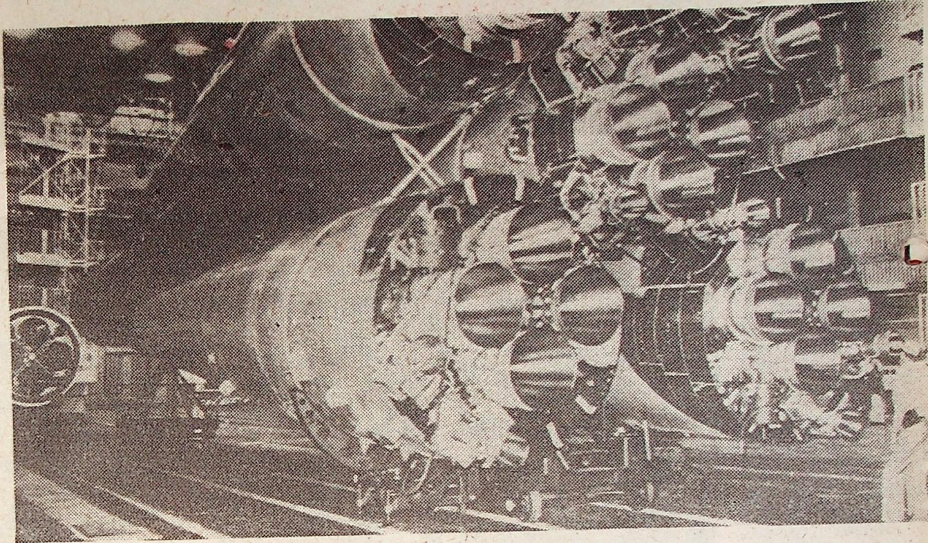
Człon napędowy radzieckich statków kosmicznych na stanowisku przygotowawczym.
