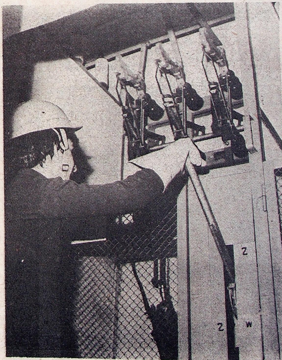
Za chwilę Andrzej Dola zamelduje: — Kabel 230 odłączony, wyłączony, uziemiony...
