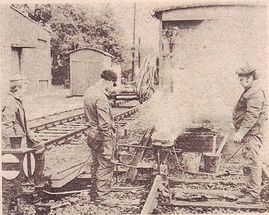
Za pomocą spawania termitowego powstają szyny bezстыkowe. Przy pracy spawacze: Wacław Jakubiak, Marian Marciniak i Andrzej Paluch.
