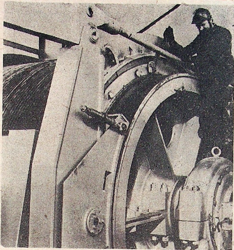
Hala maszyny wyciągowej. Przygotowanie do uruchomienia wyciągu. Maszynierę konserwuje Włodzimierz Romatowski.
