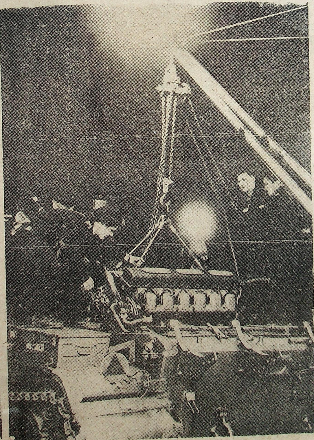
Żołnierze, remontowcy wymieniają silnik w uszkodzonym transporterze opancerzonym.
