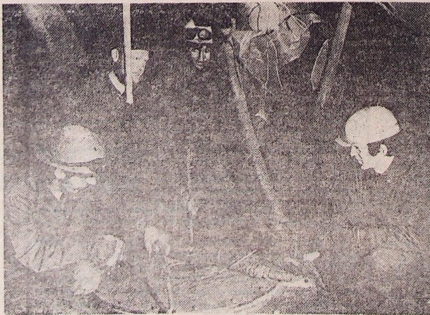
Remont pieca zawieszinowego w HM „Głogów-2”. Brygada młodzieżowa ZREM: Tadeusz Wiertelak, Tadeusz Kobylka, Stanisław Mędrala i Czesław Leśniak (brygadziści) w czasie montażu palników szybu reakcyjnego.
