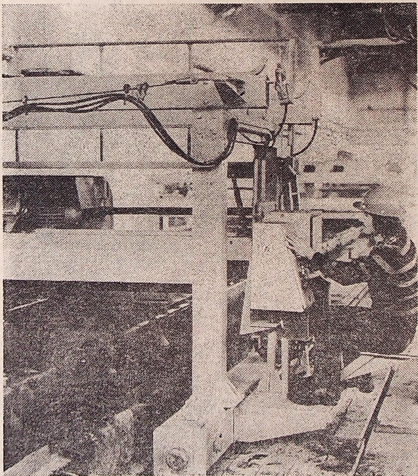
Leszek Dyk obsługuje nowoczesną betoniarkę na linii produkcji płyt. Fot. Krzysztof Raczkowiak
