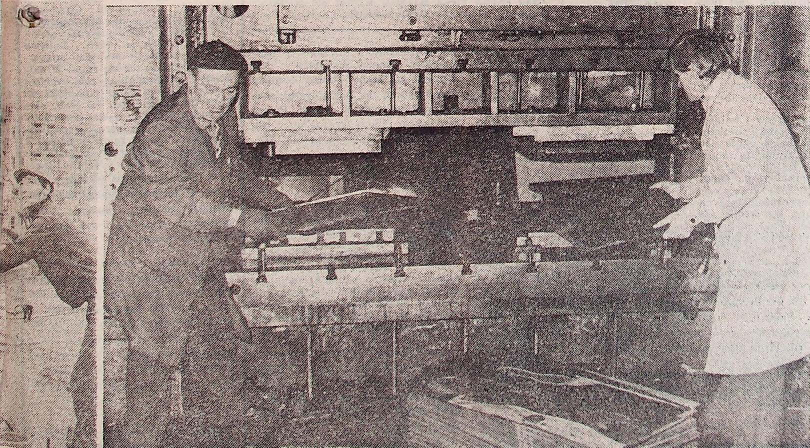
Tłocznia Fabryki Wyrobów Metalowych w Jaworze. Tutaj walcowano i wykrawano tylne ścianki do dodat- kowych kuchni węglowych „Magda”.
