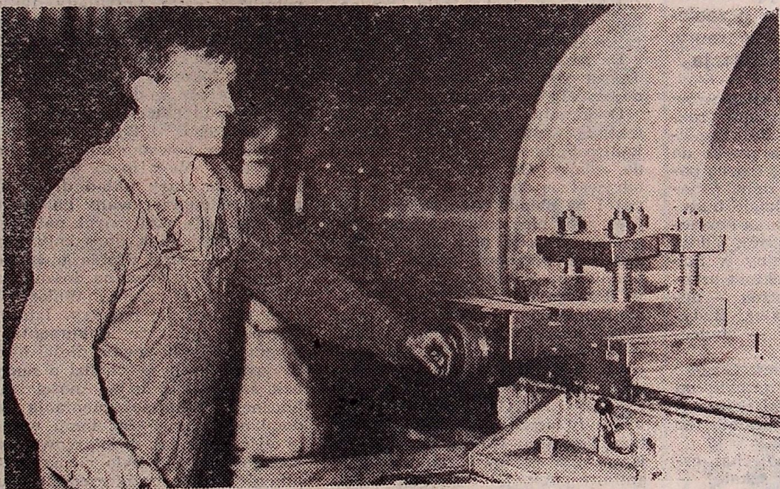
Obróbka powierzchni zewnętrznej i wewnętrznej walca wymaga dużej precyzji i wprawy. Edward Kehle ma w tej mierze doświadczenie.
