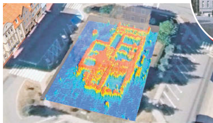
Wyniki prospekcji georadarowej
