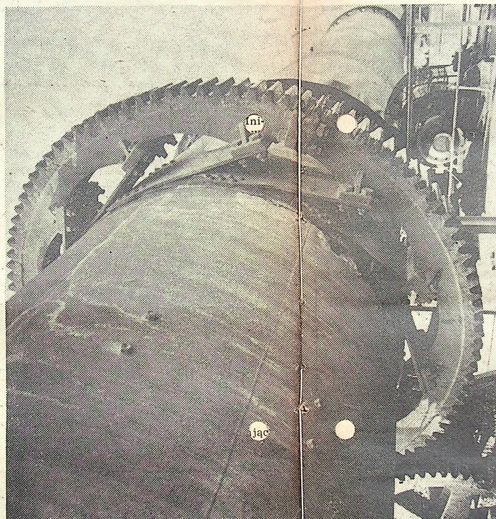
Fragment potężnego pieca obrotowego do produkcji cementu.
