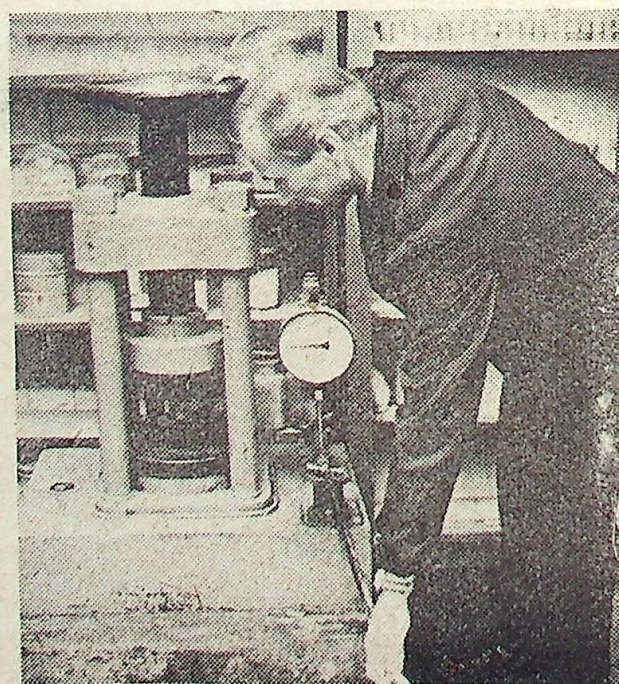
Nowe materiały budowlane muszą przejść dokładną próbę wytrzymałości. Przeprowadza ją laborant Bolesław Opala.
