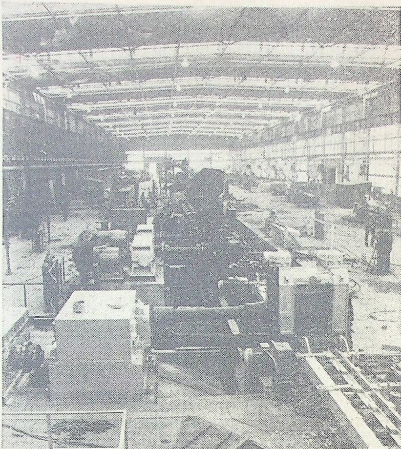
W Szopienicach (woj. katowickie) kończy się budowa walcowni brzdowej miedzi. Na zdjęciu: Montaż maszyn na linii walcowniczej.
