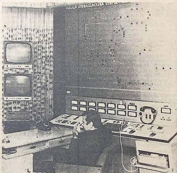
Lech Adamiak obsługuje nowoczesną dyspozytornię Wydziału Ciągłego Odlewania Miedzi w hucie „Legnica”.
