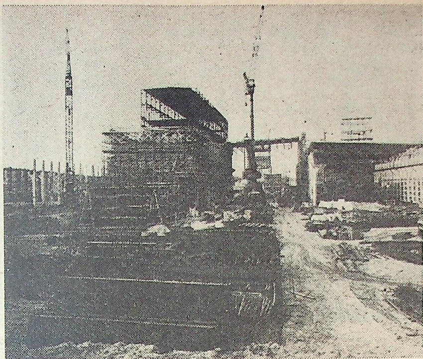
Na placu budowy zakładu przeróbki mechanicznej ZG „Rudna”. Fot. Tadeusz Matkowski
