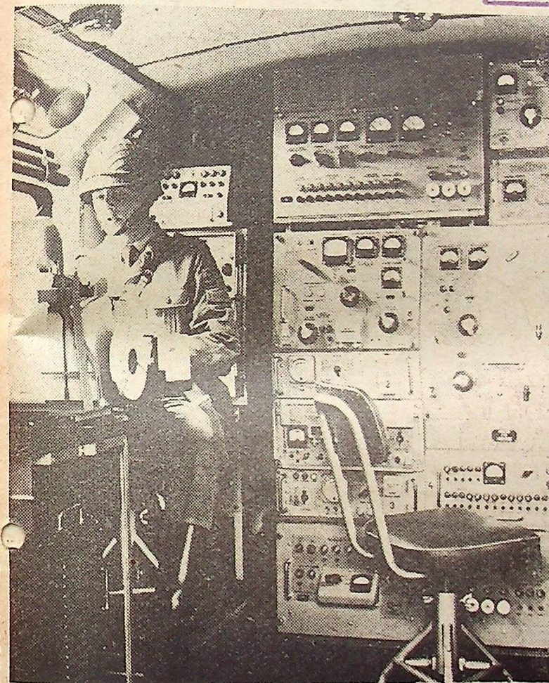
Pracę nowoczesnej, zamontowanej w samochodzie radiostacji kieruje młodszy chorąży Michał Rusinek — prymus szkoły w roku 1971.
