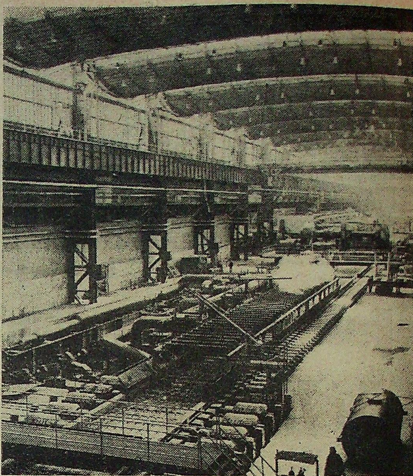
Walcownia blach grubych w Hucie im. Bieruta w Częstochowie. Fot. CAF — Jakubowski
