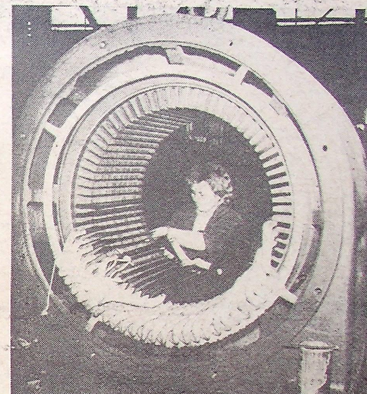
Przewijanie uzwojenia silnika elektrycznego o mocy 500 KW wymaga sprawności i precyzji kobiecych rąk... Teresa Mossur — jedna z niewielu specjalistek od silników...
