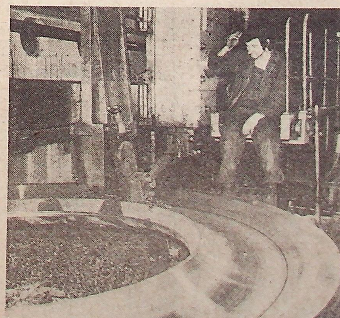
Toczone przez Zbigniewa Kasjana potężne pierścienie młyna kulowego są cennym towarami dla zakładów przeróbki mechanicznej rudy miedzi.
