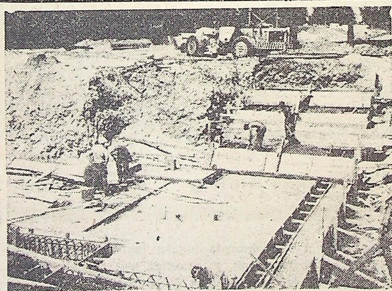
Warszawa. Przestrzeń między mostem Śląsko-Dąbrowskim, a Cytadłą. Jedenastu górników z Przedsiębiorstwa Budowy Kopalni Rud Miedzi w Lubinie buduje cztery podziemne przejścia dla pieszych pod Wisłastradą. Tempo prac i ich organizacja zwracają uwagę przechodzących warszawiaków. Ich praca to dobra propaganda zdolności i możliwości miedzianego zagłębia.
