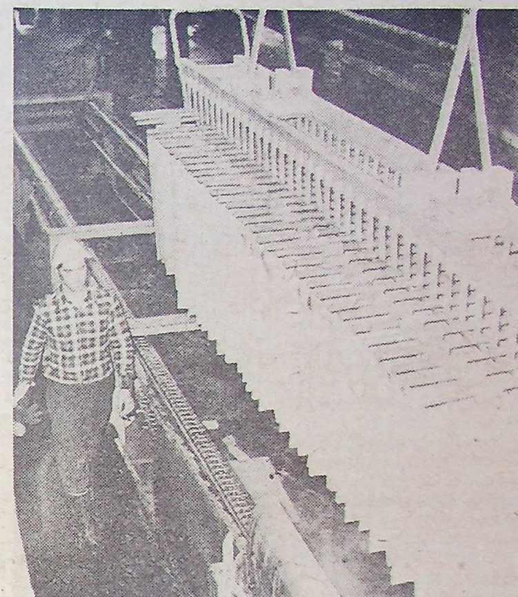
Za chwilę suwnicowy umieści zespół katod w urządzeniu do mycia gorącą wodą.
