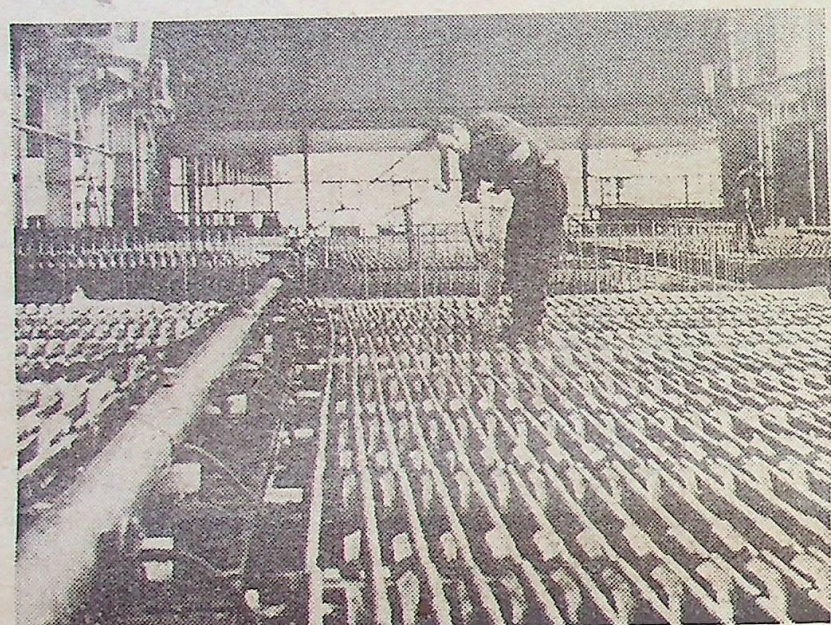
Usuwanie zwarć i zarazem kontrola katod.
