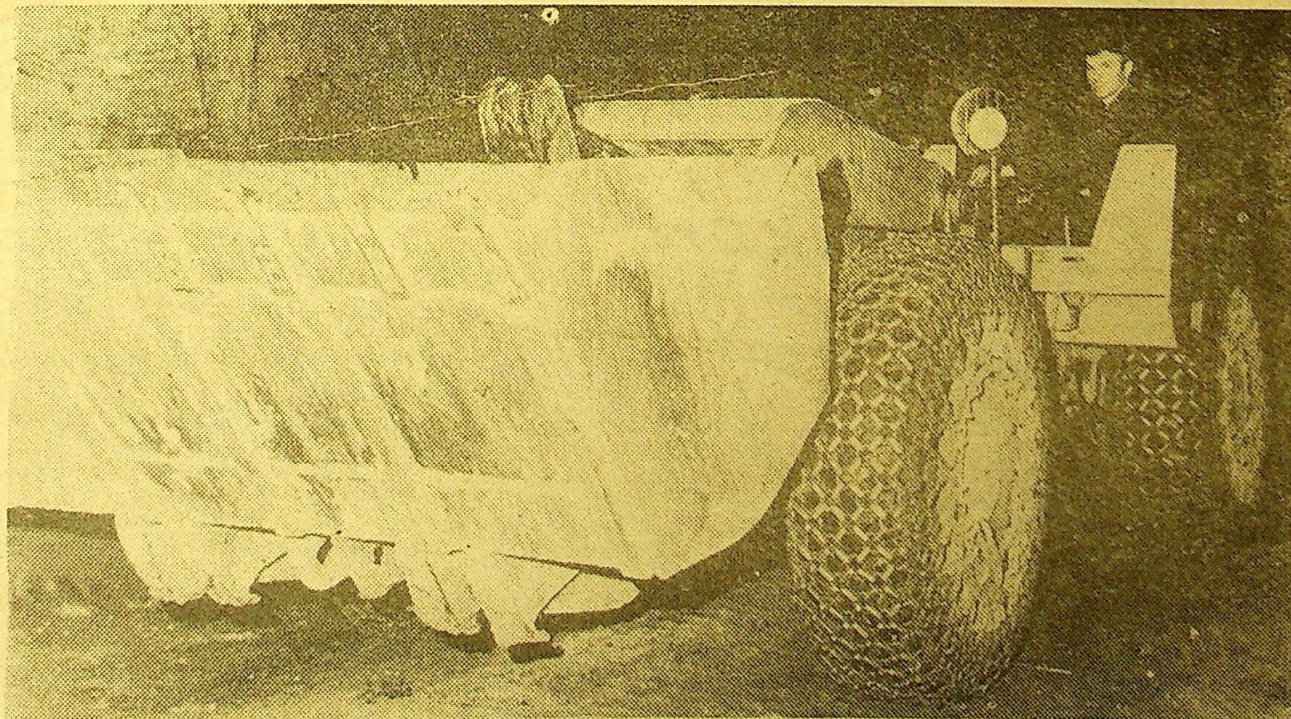
Wóz odstawczy produkowany przez firmę „Joy”, popularnie zwany „dżojem”, odstawia jednorazowo z przodka 12 ton rudy
