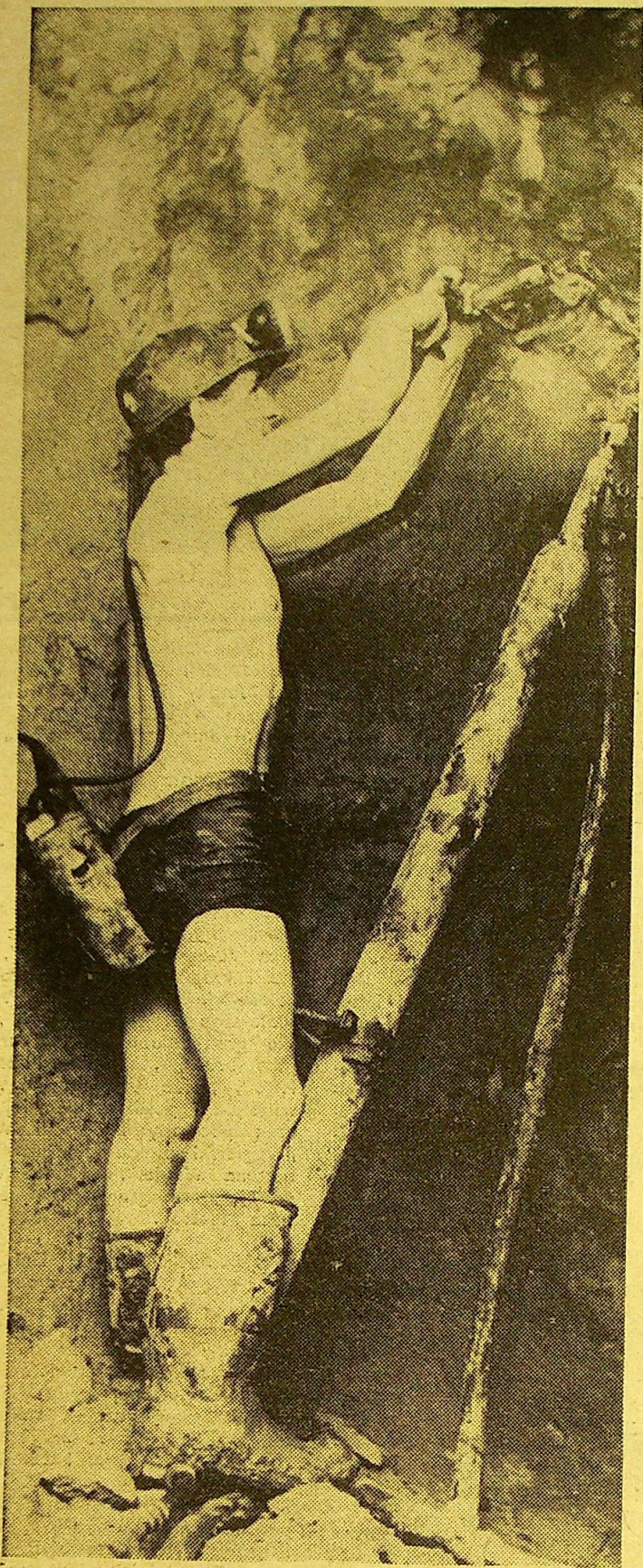
Kotwienie ręczne wymaga wiele wysiłku, jest czasochłonne i uciążliwe dla górnika.
