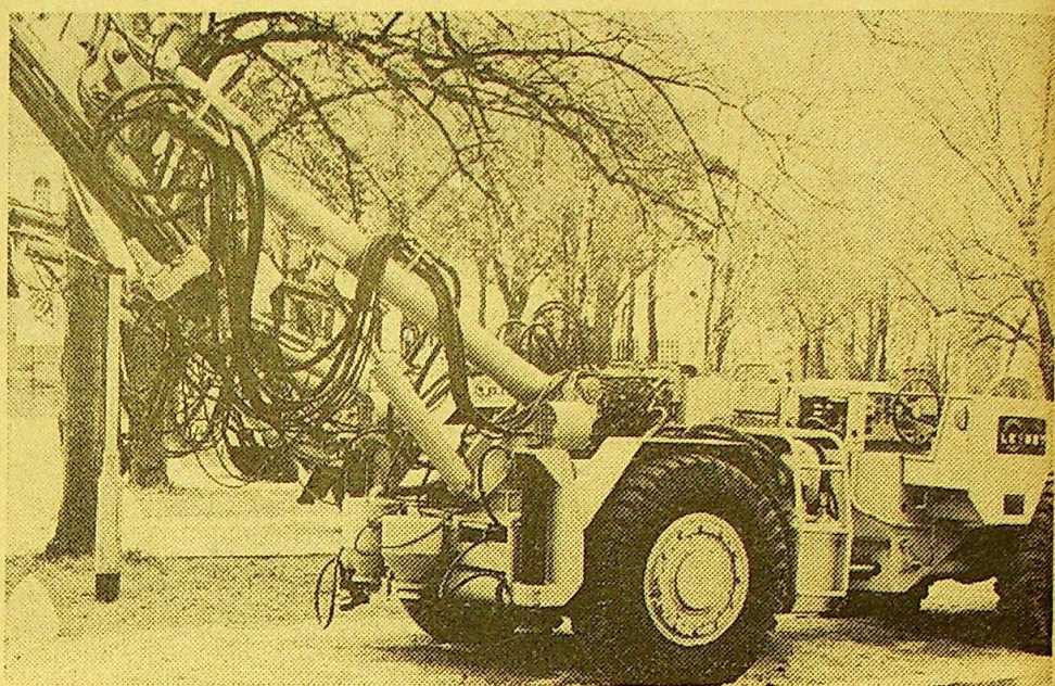
Nowe maszyny do kotwienia produkowane przez legnicki „Legmet”, wyposażone w importowane układy hydrauliczne i silniki produkowane w kraju na licencji „Leylanda”, należą do najnowocześniejszych maszyn tego typu używanych w górnictwie.
