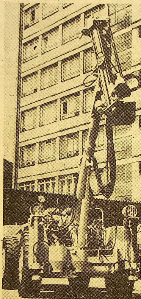
Hydrauliczna kotwiarka produkowana w „Legrecie”. Fot. K. Kiefer
