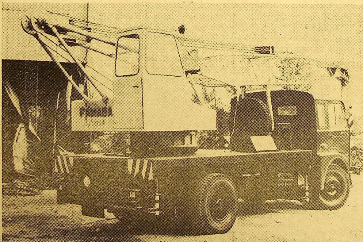
W tym roku z taśmy produkcyjnej zjechało kilkadziesiąt żurawi „Hydros-10”. Konstruktorzy spoza zakładu pokpiłi sprawę z ogranicznikami wysięgu dźwigi nie mogły być sprzedane w obawie przed wywróceniem się. Na miejscu naprawiono ten błąd i część „Hydrosów” trafiła już do odbiorców w kraju i za granicą.
