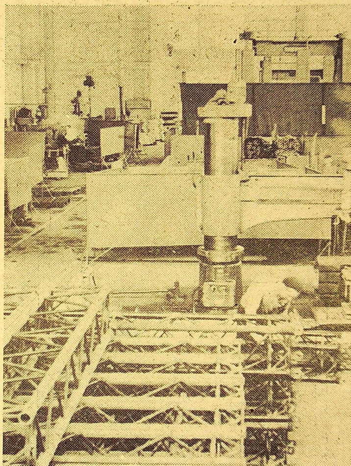
Widok ogólny hali montażowo-spawalniczej.
