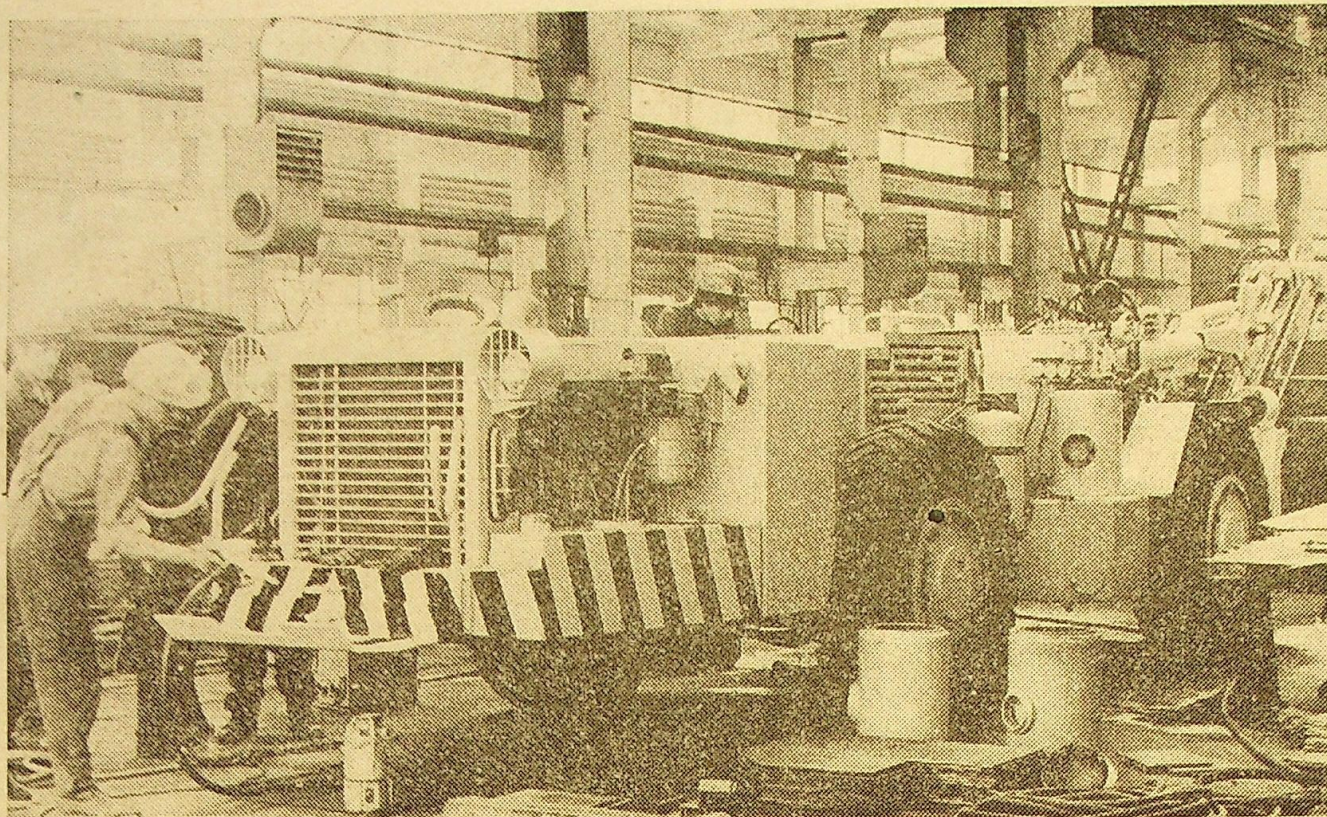
Na wydziale konstrukcyjnym ostatnie prace przy samojezdnym wozie do kotwienia.
