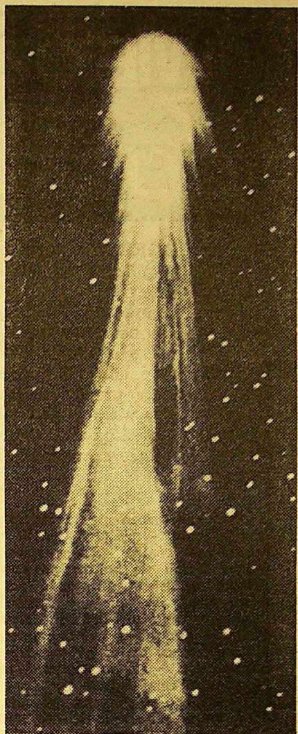
Zdjęcie astronomiczne jednej z „włochatych gwiazd”. Widzimy głowę komety i efektywny strzępiasty warkocz.
