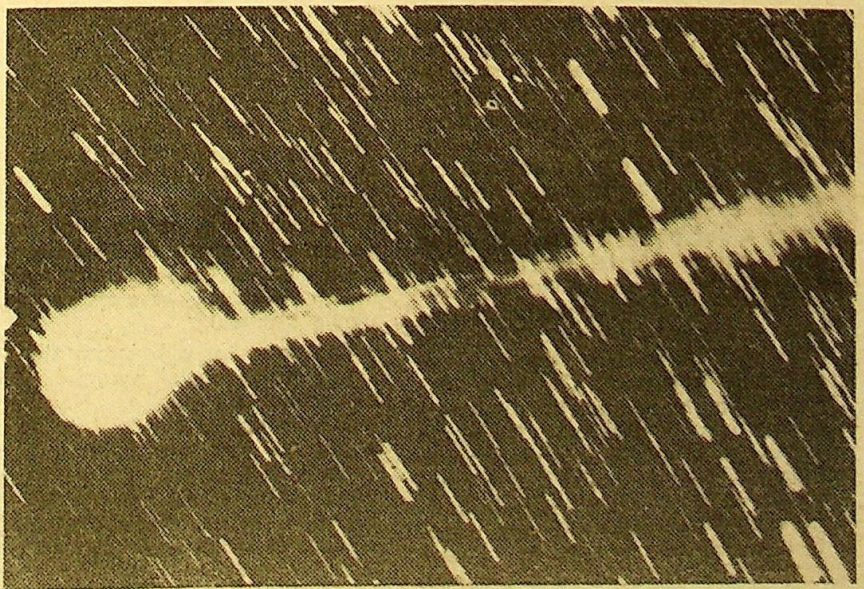
Zdjęcie komety Burnham — 1960 — II wykonane w obserwatorium astronomicznym Lowell w Flagstaff (USA). Astronomowie zaobserwowali, iż kometa ta macha swym ogonem długości 2,896 tys. km raz na 4 dni. Jest to pierwsza kometa zachowująca się tak dziwnie, zaobserwowana przez astronomów.
