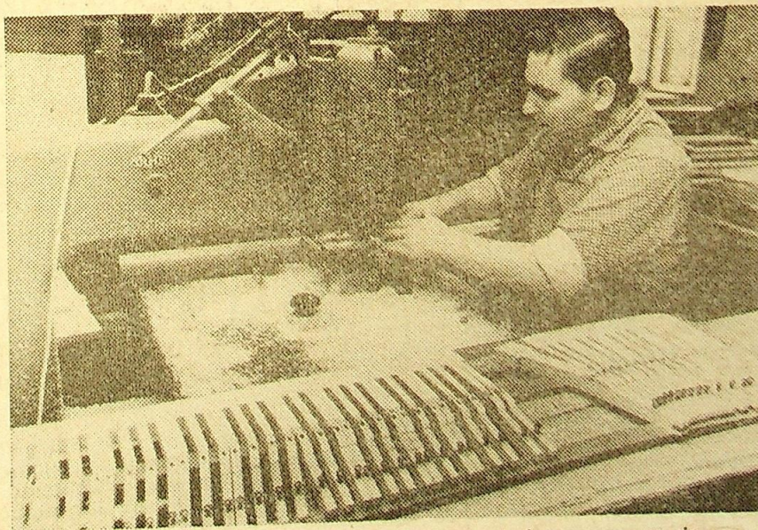
Czynność, którą wykonuje Czesław Halter fachowo nazywa się frezowaniem białych klawiszy.
