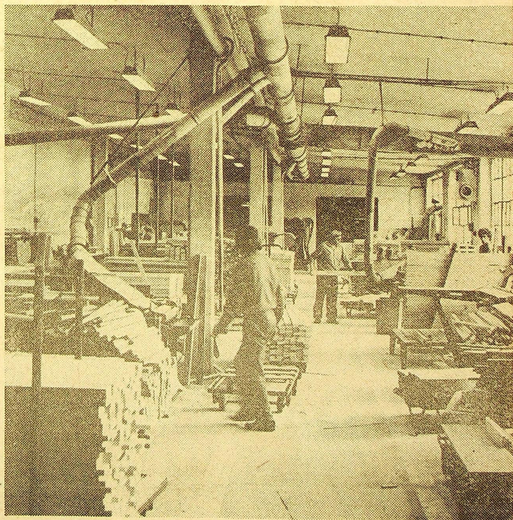
Tutaj, w stolarni, powstają wszystkie drewniane części pianina.
