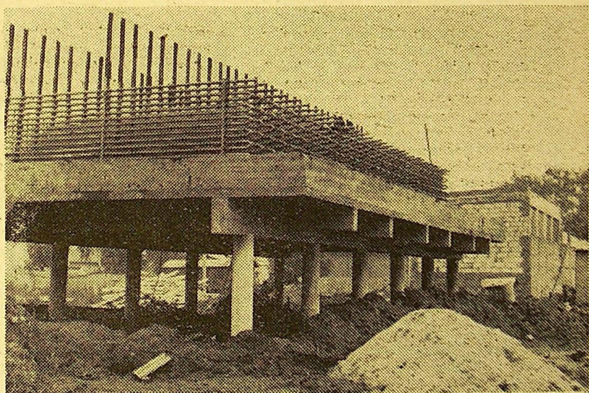
Jednym z najważniejszych obiektów wchodzących w skład lodowiska jest urządzenie skraplające.
