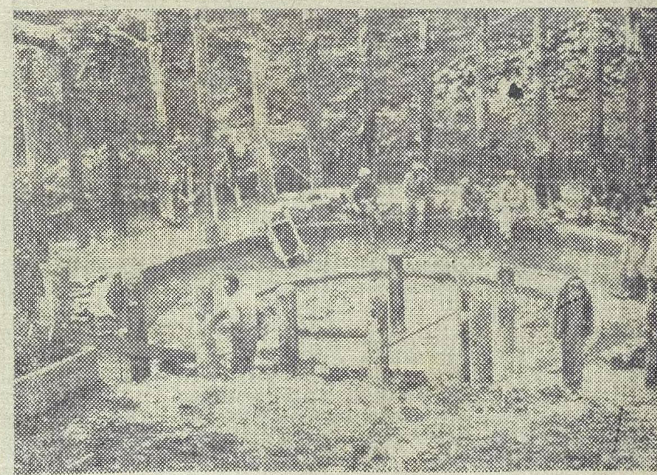
Trwa budowa tak zwanej głowicy mroźniowej pod szyb wentylacyjny — zachodni.
