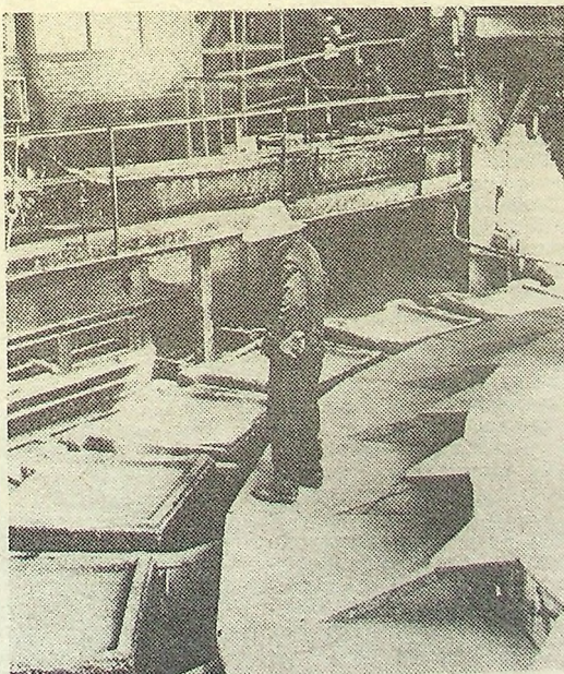
Na tej zmianie nie było wytopu. Sprawdzano, oczyszczano i wyważano formy do odlewania anod na maszynie karuzelowej.
