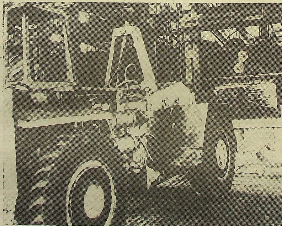
Strawa dla pieca — wsad. Samojedźny pojazd zwany wsadzarką obsługiwany jest przez Andrzeja Łukasiewicza.
