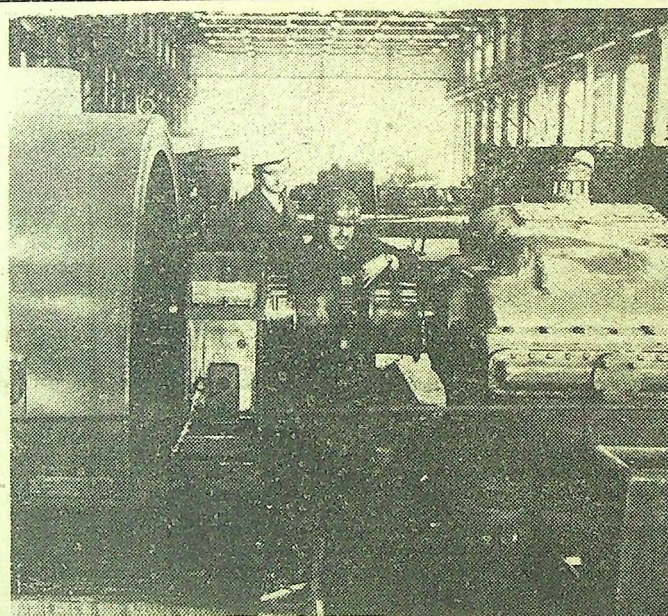
Kompresorownia, montaż agregatu.
